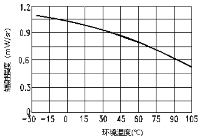
图六：相对辐射强度和环境温度关系曲线
