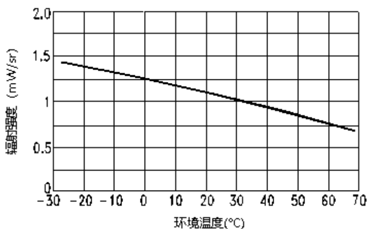
图六：相对辐射强度和环境温度关系曲线
