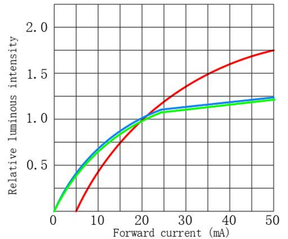
相对光强与正向电流特性 Relative Luminous VS Forward Current
