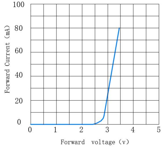
伏安特性 Volt ampere characteristic
