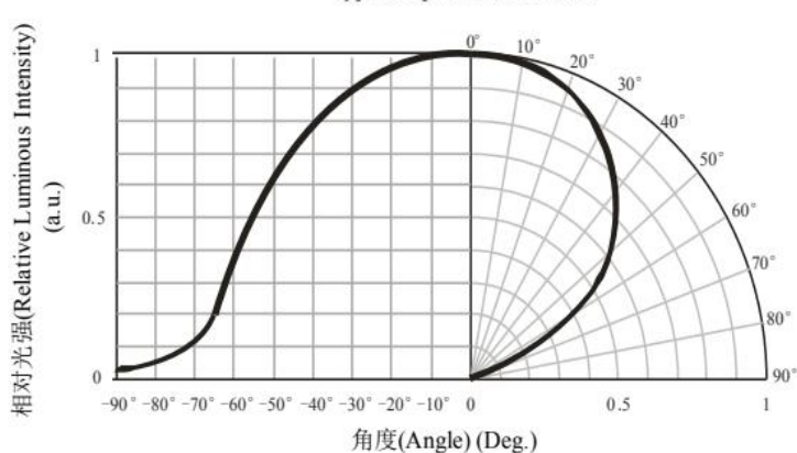
光强分布特性曲线 Typical Spatial Distribution
