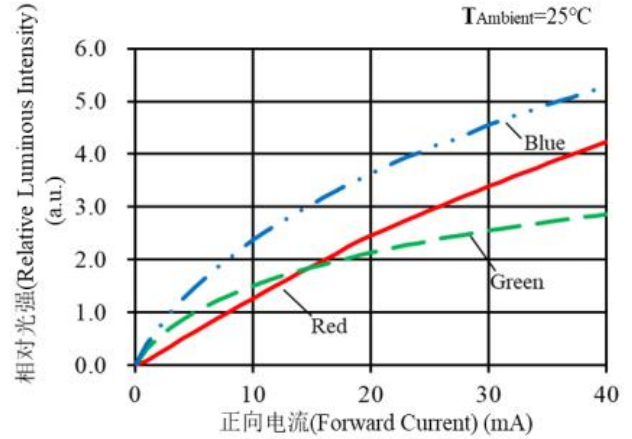
相对光强与正向电流特性 Relative Luminous Intensity VS Forward Current T_{Ambient}=25^{\circ}C
