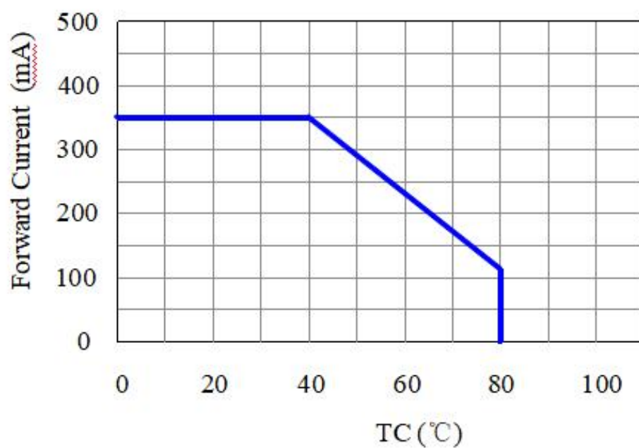
环境温度 VS. 正向电流关系图
