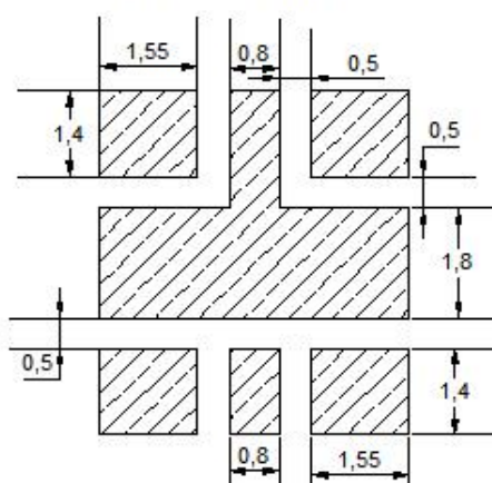
建议焊盘图
