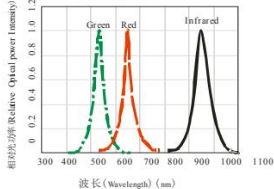
光谱分布特性曲线 Relative Spectral Distribution
