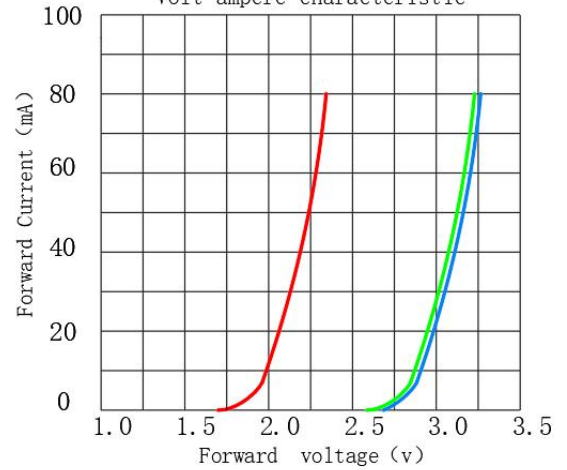
伏安特性 Volt ampere characteristic
