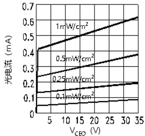
图六：光电流VS VCE曲线
