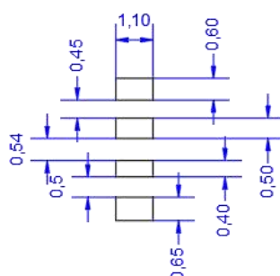
建议焊盘图 仅供参考
