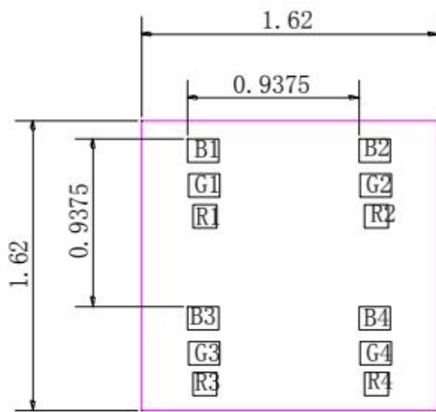
灯面正视图
