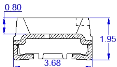
侧面图
