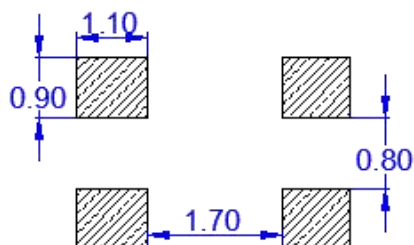
建议焊盘图
