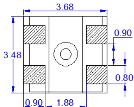
建议焊盘图
