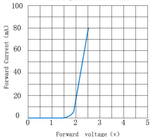
伏安特性 Volt ampere characteristic
