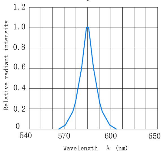
光谱分布曲线 Relative Spectral Distribution
